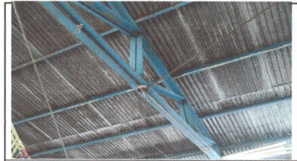
FOTO 6: Instalación de lámina troquelada aluzinc
